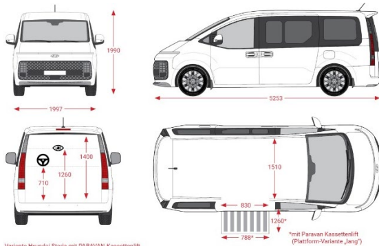
Variante Hyundai Staria mit PARAVAN-Kassettensitz
